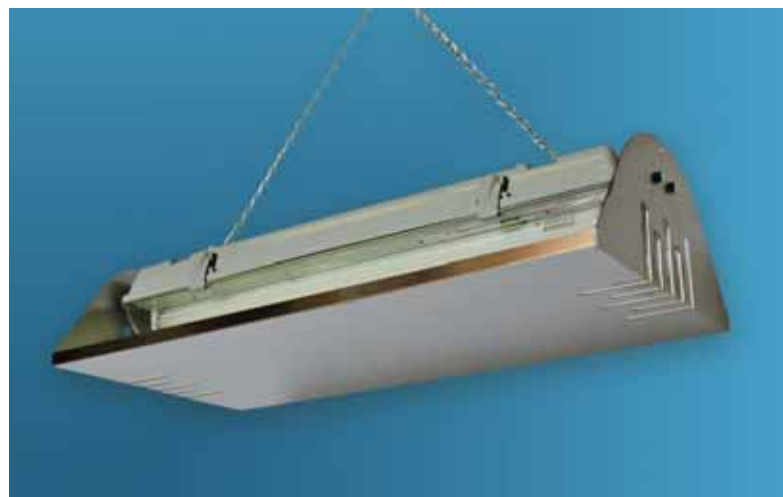
Exterminador de insectos con trampa adhesiva. Estanco IP65. Para ambientes con alto nivel de humedad. Posición suspendido, material acero-inox.
